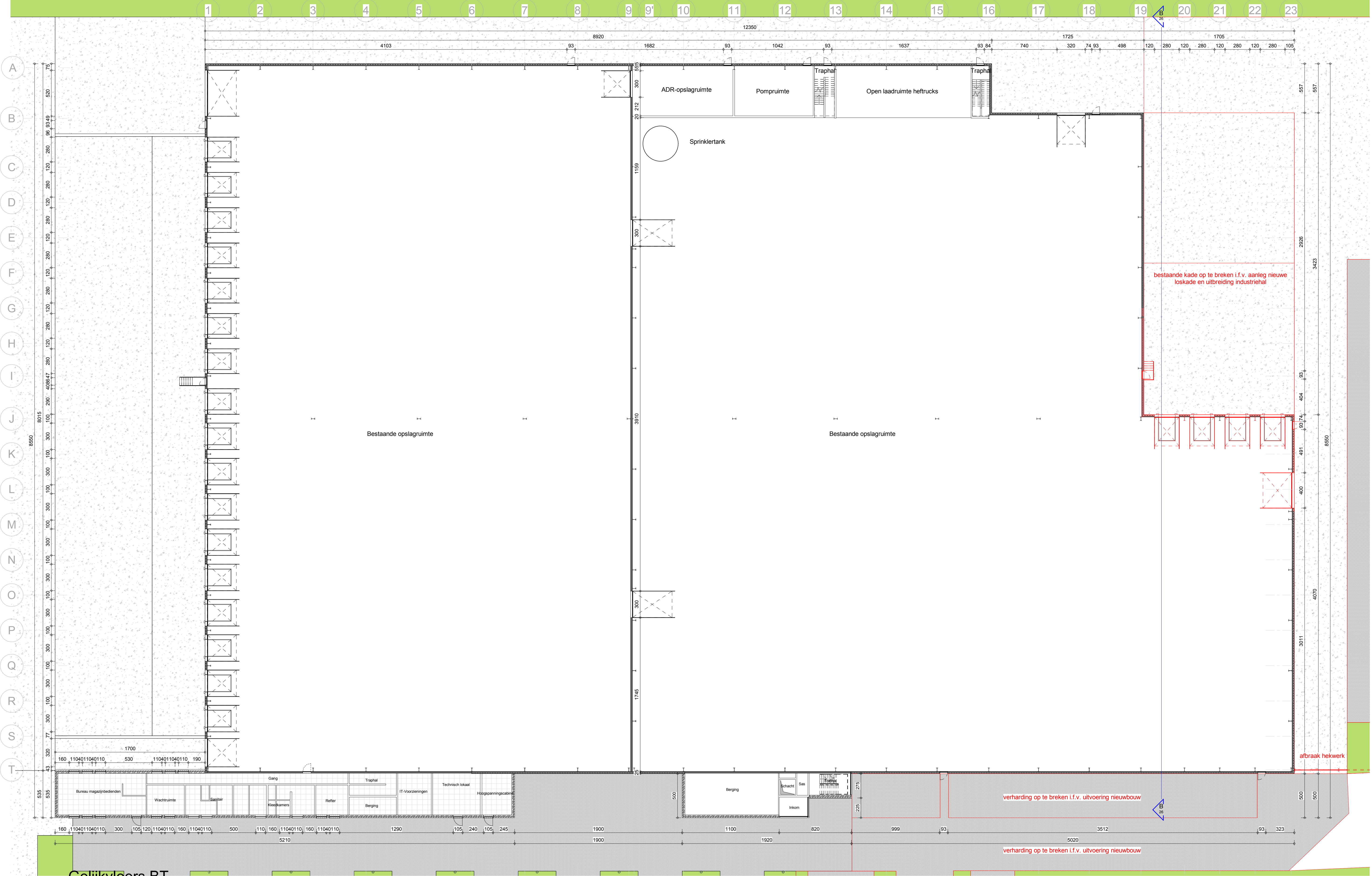
Gelijkvloers BT 1 : 200
