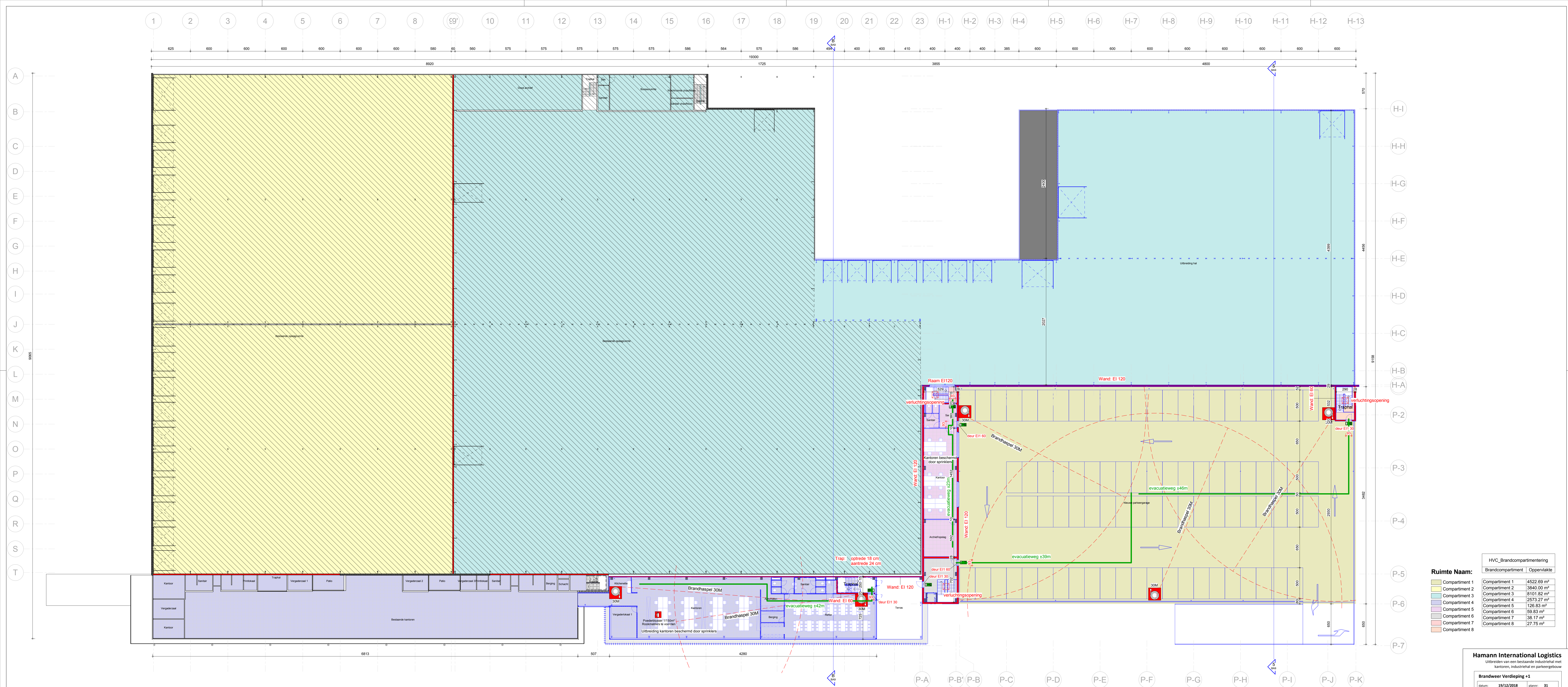
Verdieping +1 - brandweer 1 : 200
