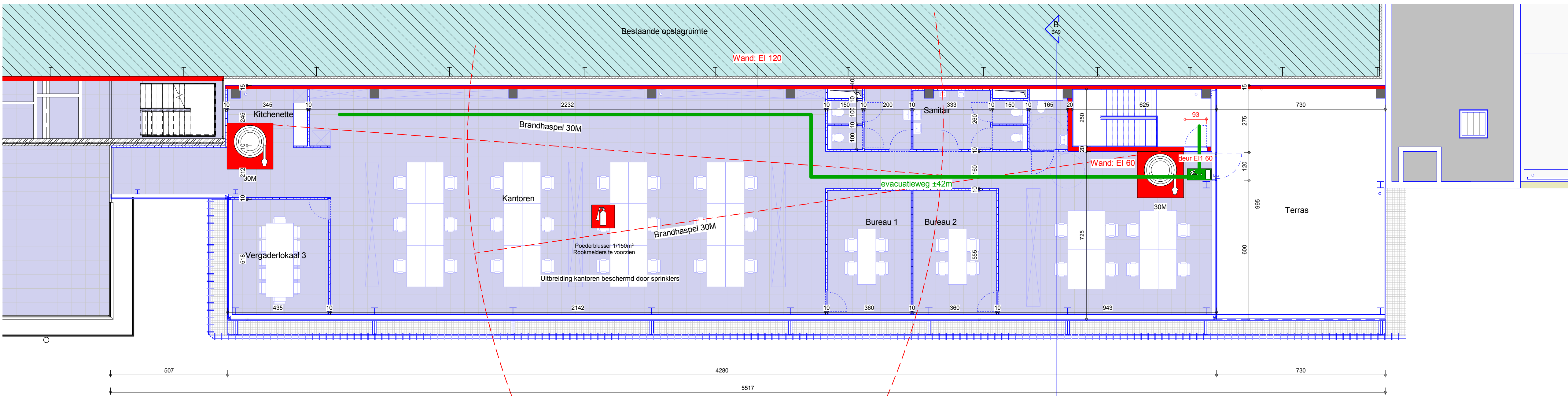
Detail Verdieping +2 NT Brandweer
