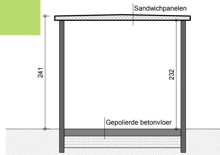
Doorsnede 1 : 50
