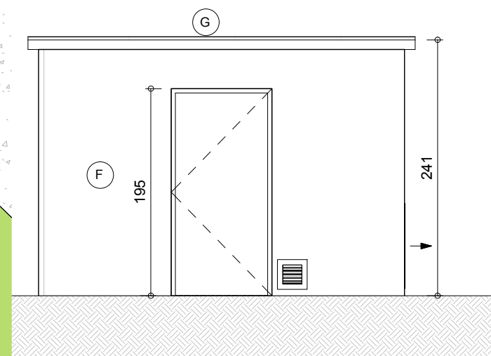
Achtergevel 1 : 50
