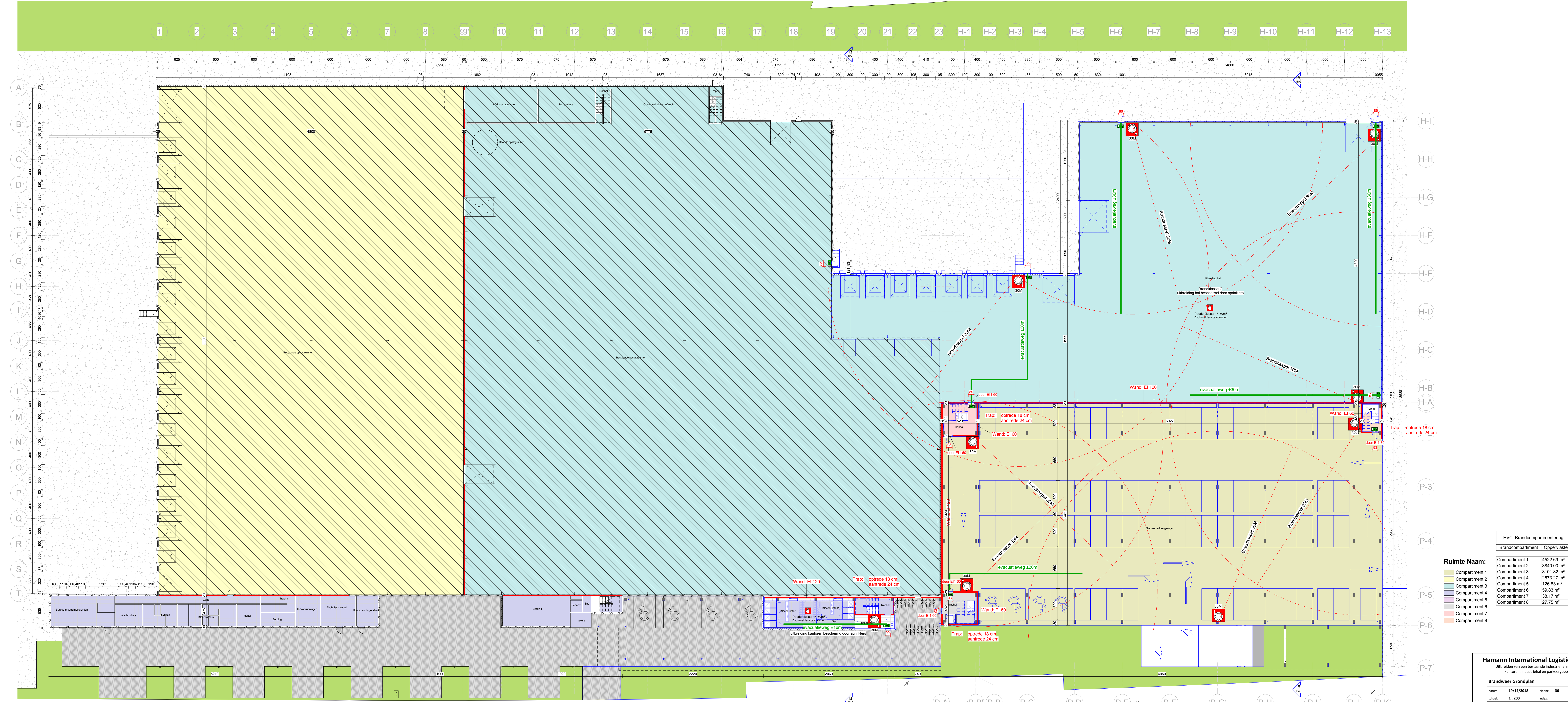
Gelijkvloers - brandweer 1 : 200
