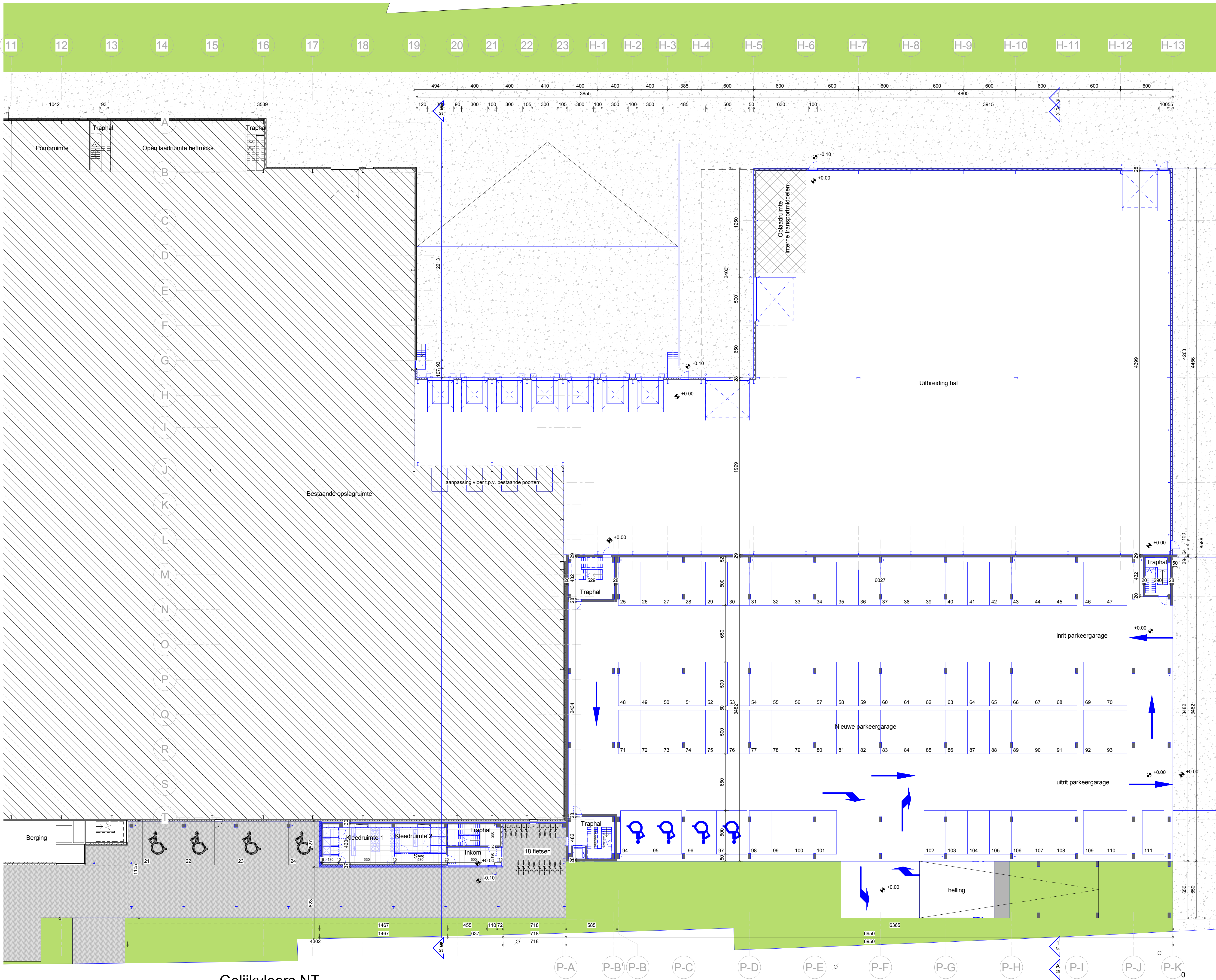
Gelijkvloers NT 1 : 200
