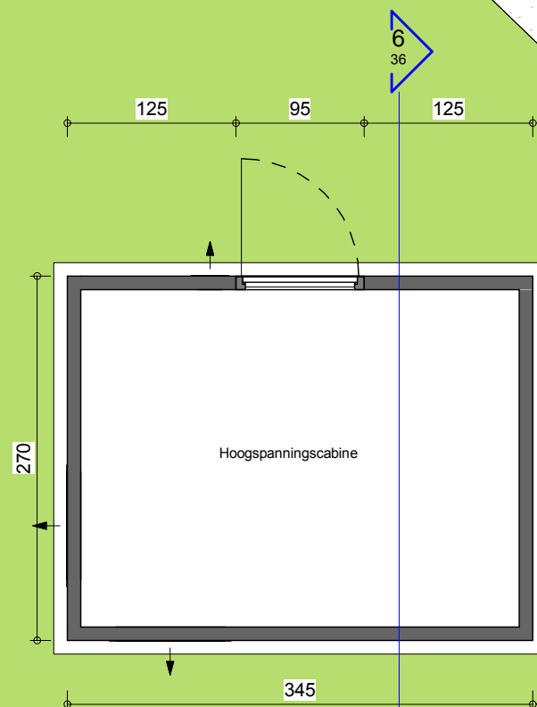
Grondplan 1 : 50
