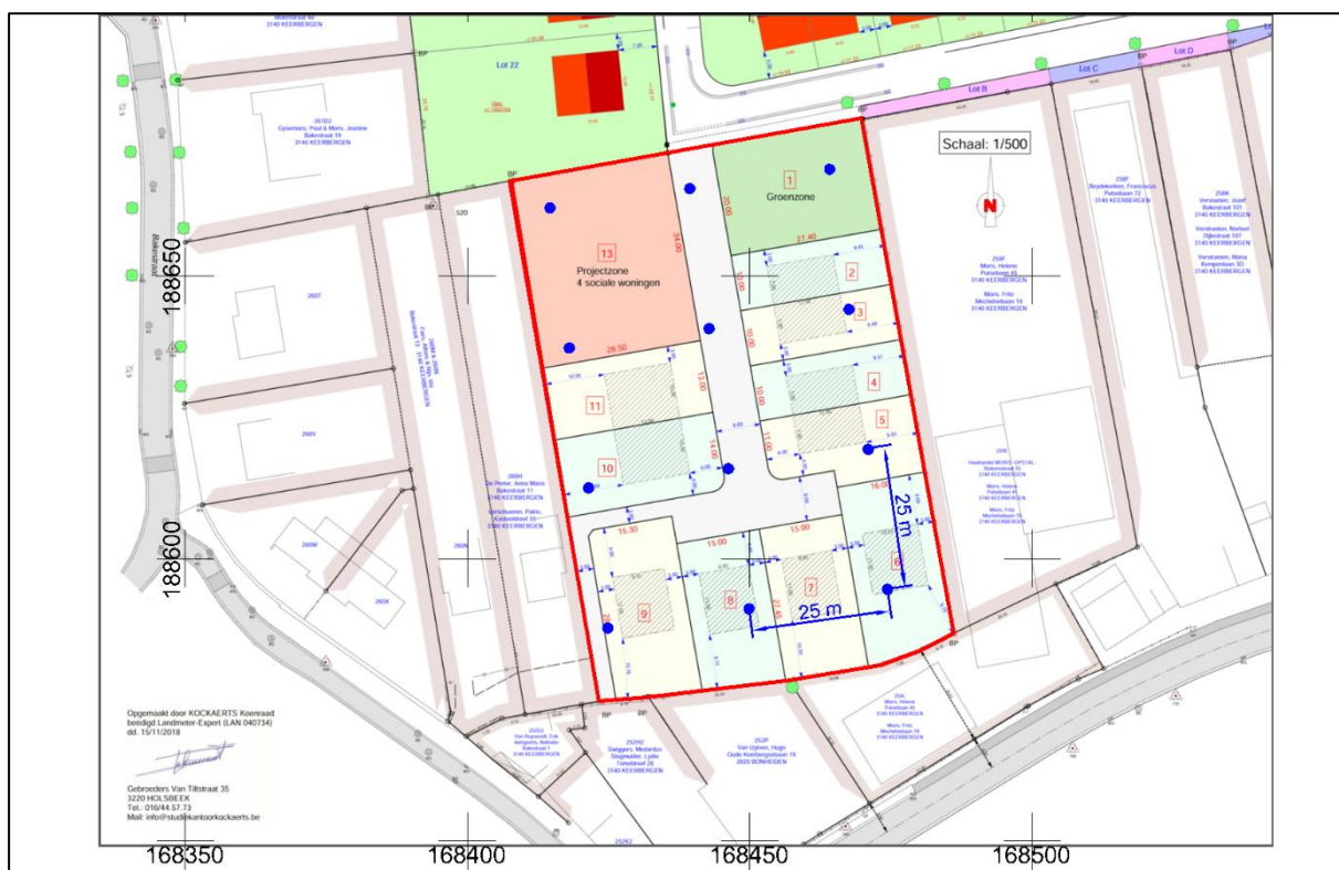
Afbeelding 8: voorstel van de boringen op de geplande werken
