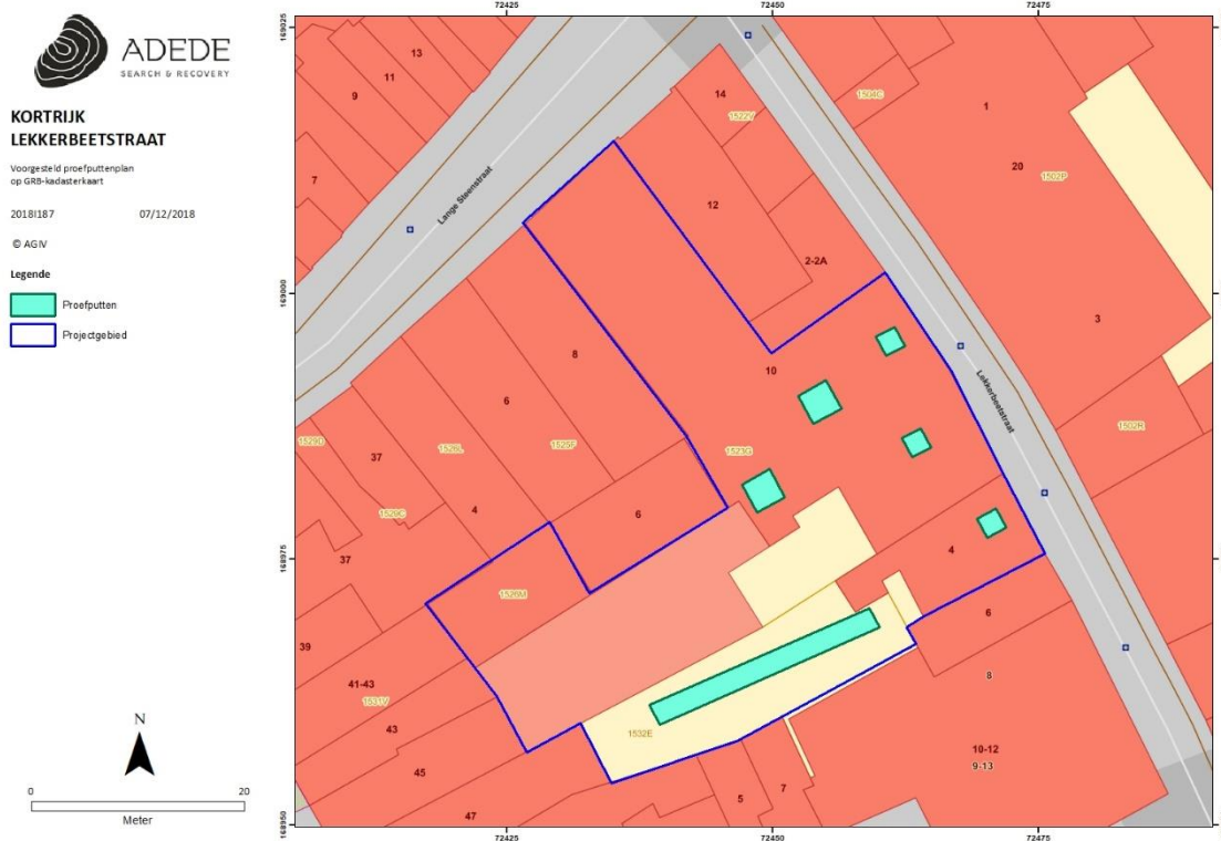
Figuur 1. Voorgesteld proefputtenplan op GRB-kadasterkaart.
