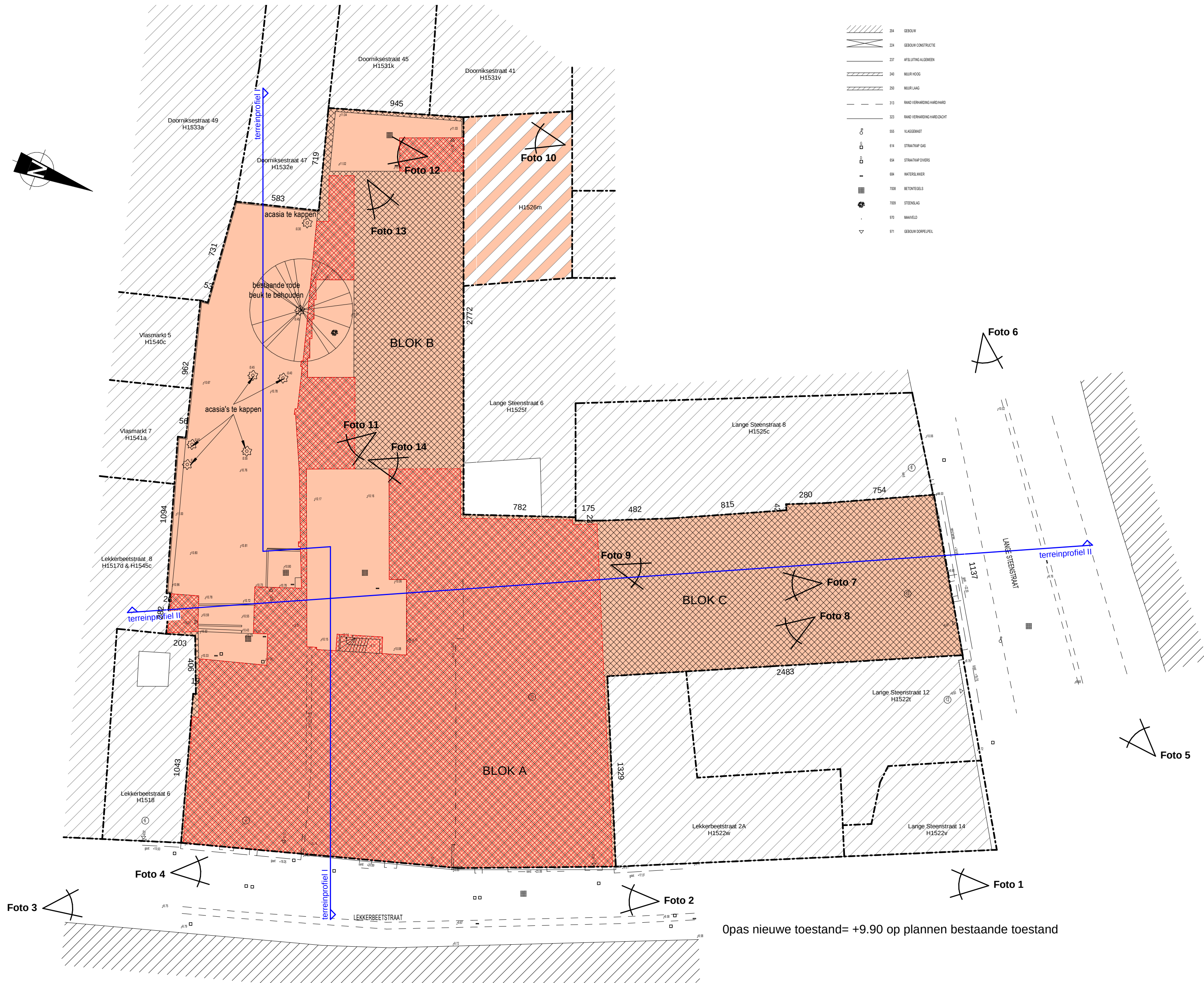
1 | Inplantingsplan - Bestaande Toestand 1:200
