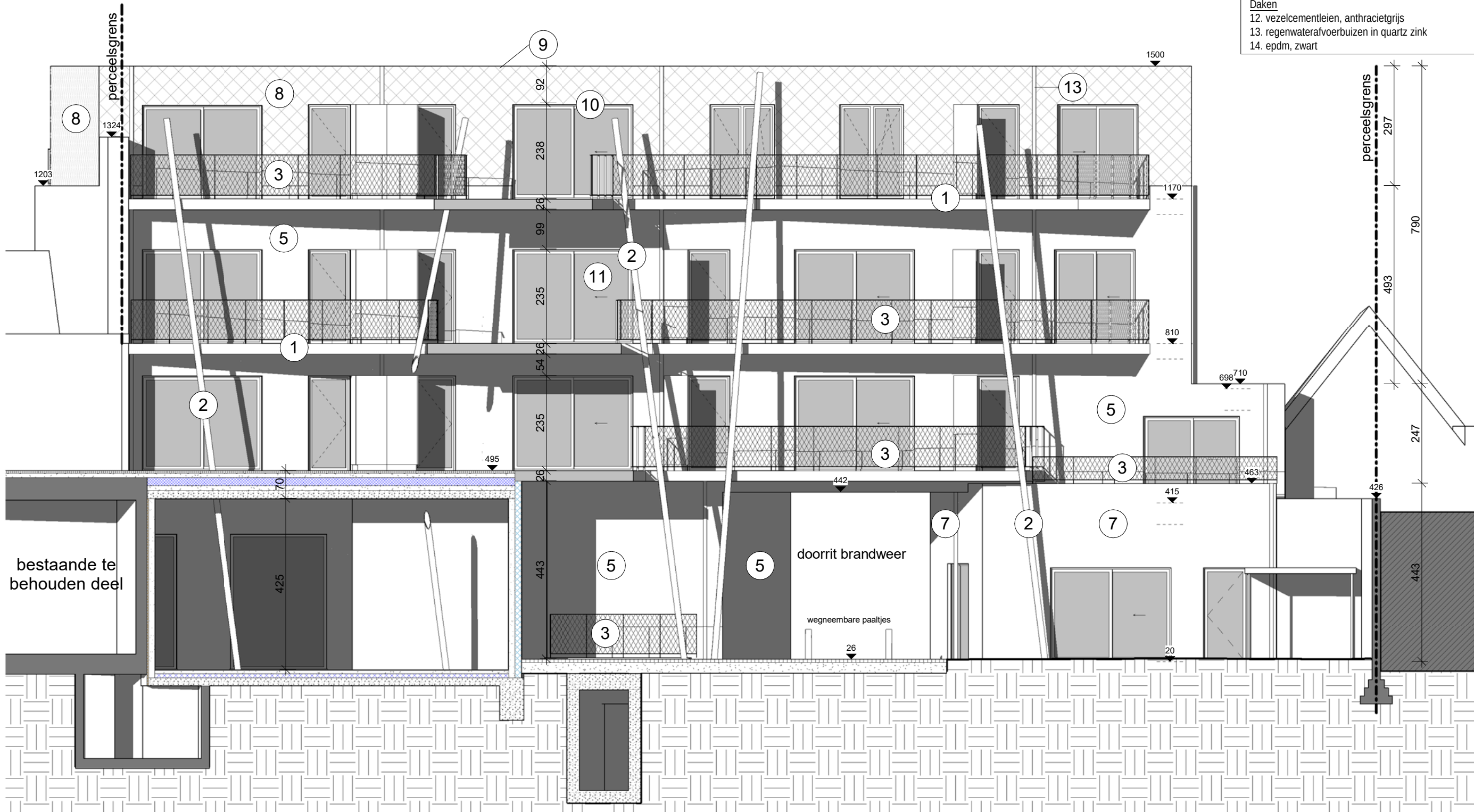
1 Achteraanzicht Blok A (Lekkerbeetstraat) - Nieuwe Toestand
