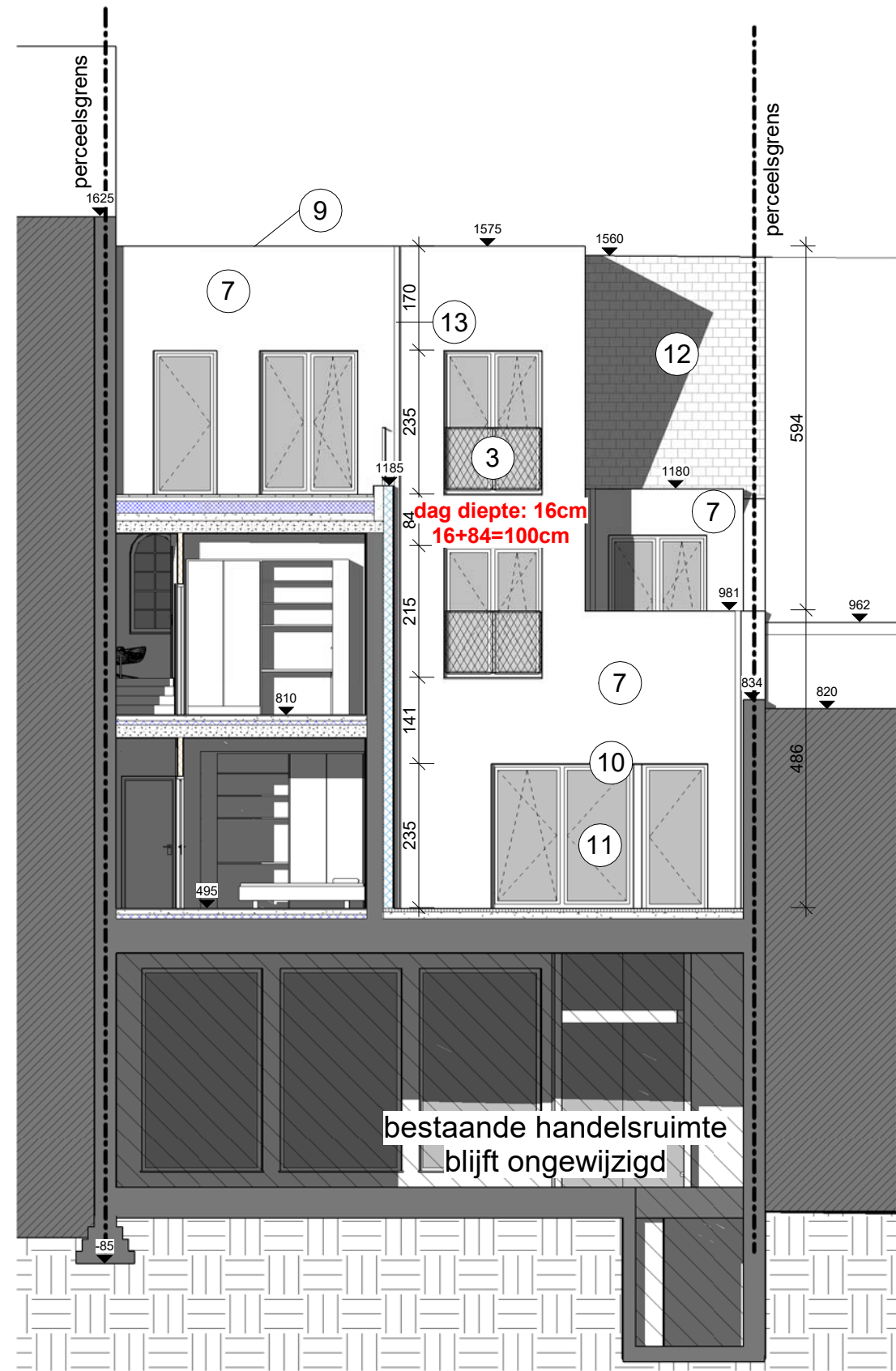
1 Achteraanzicht blok C (Langesteestraat) - Nieuwe Toestand
