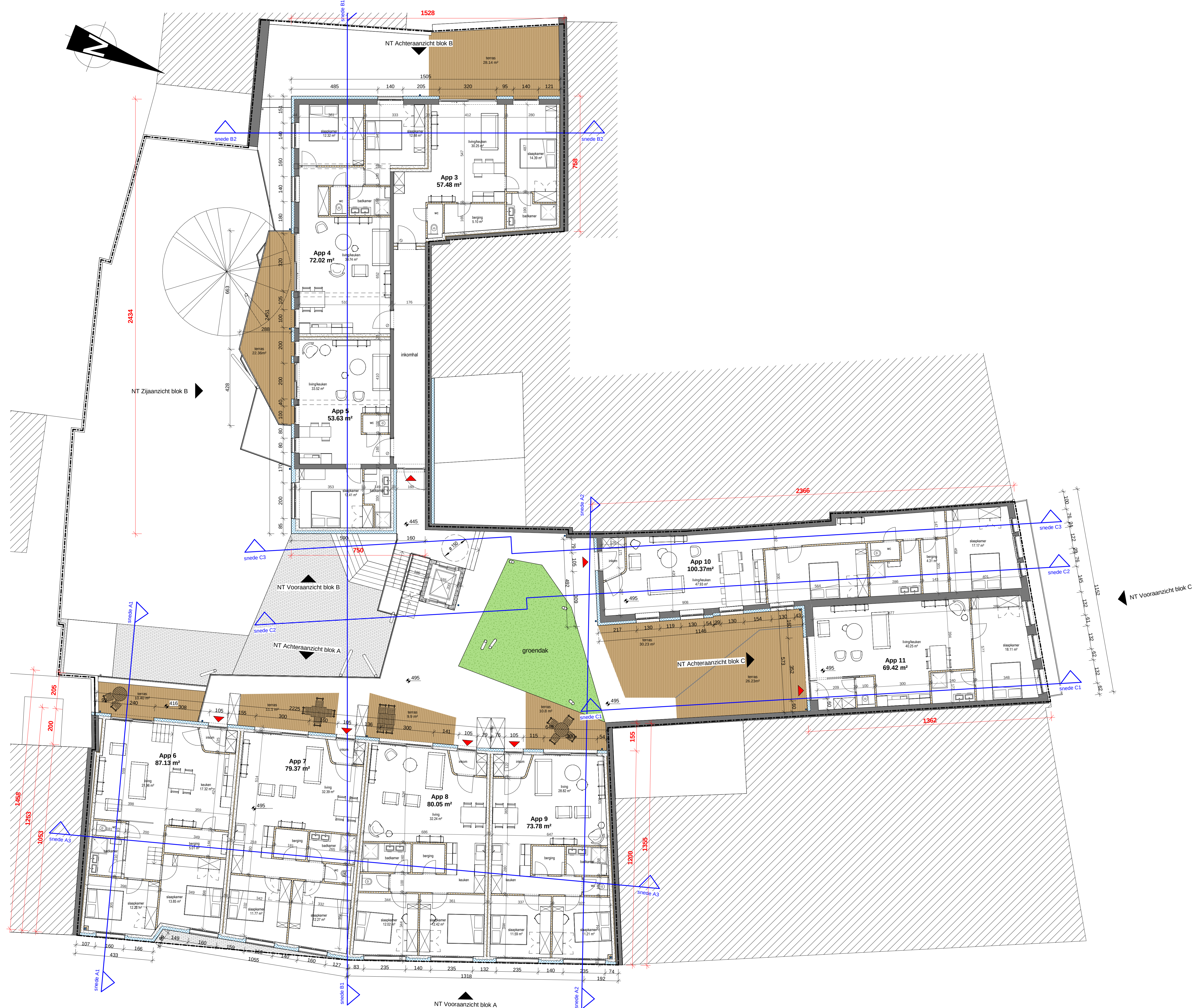
1 Eerste Verdieping - Nieuwe Toestand
