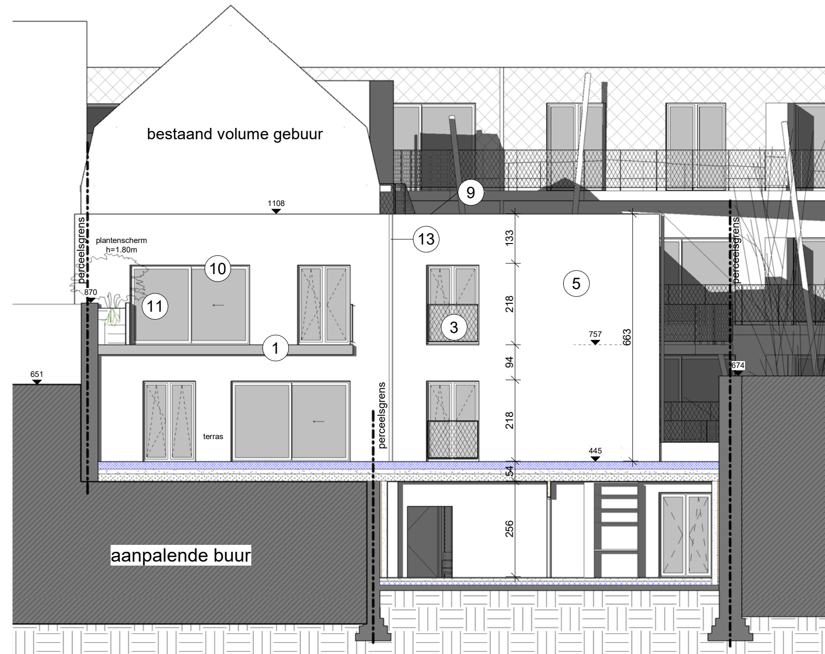
1 Achteraanzicht Blok B (Binnengebied) - Nieuwe Toestand 1:100 0 100 300cm
