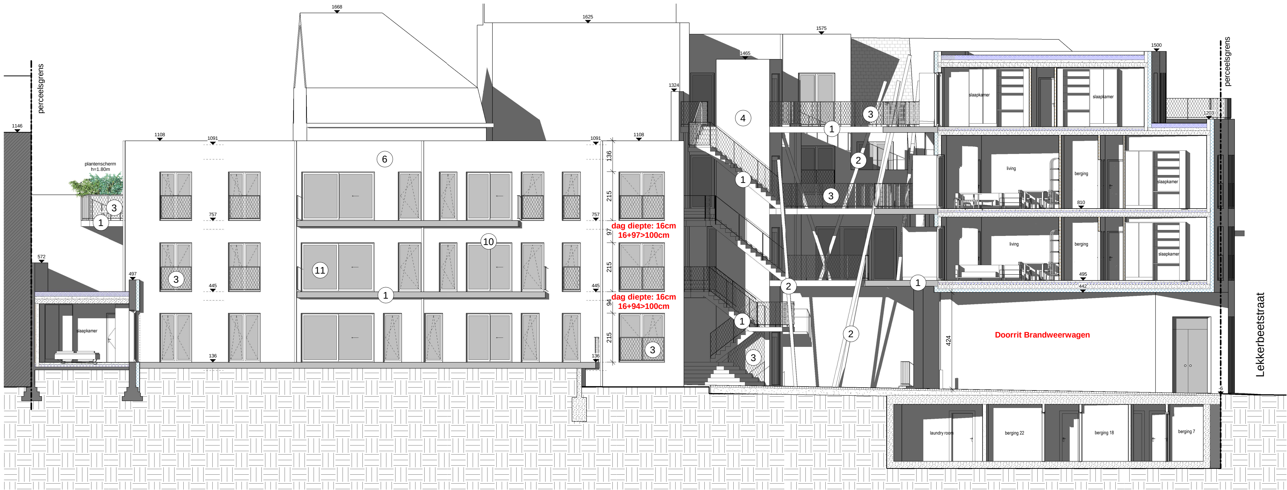
1 Zijaanzicht Blok B (Binnengebied) - Nieuwe Toestand 1:100
