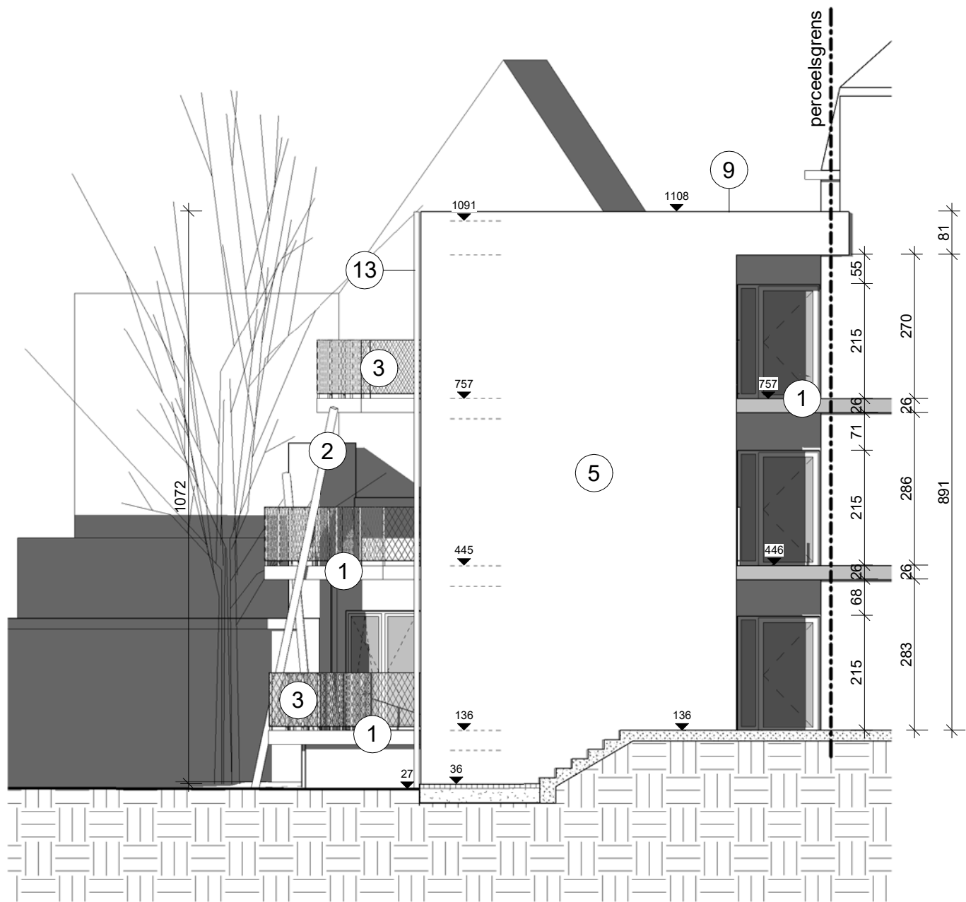
1 Vooraanzicht Blok B (Binnengebied) - Nieuwe Toestand 1 : 100
