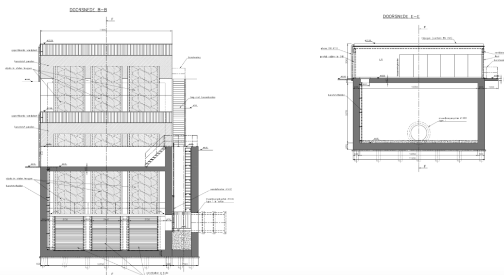
Afb. 7. Doorsnede van het nieuwe vizelgemaal in het plangebied (1/2).
