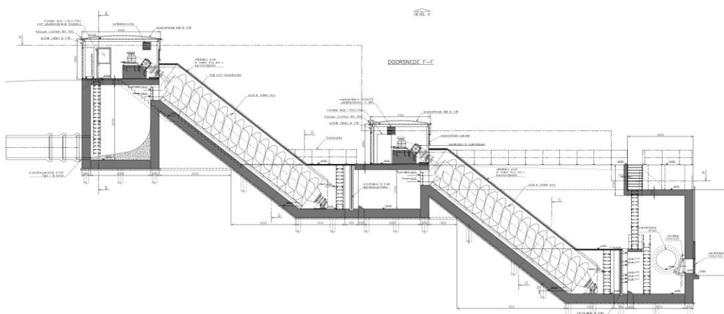
Afb. 6. Doorsnede van het nieuwe vizelgemaal in het plangebied (1/2).
