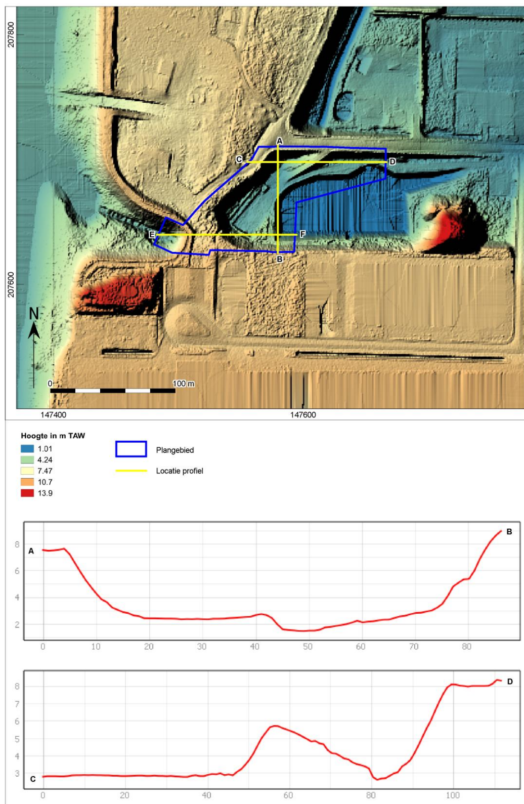
Afb. 11. Het plangebied op het Digitaal Terreinmodel Vlaanderen (DTM), inclusief profiel hoogteverloop (1/2).
