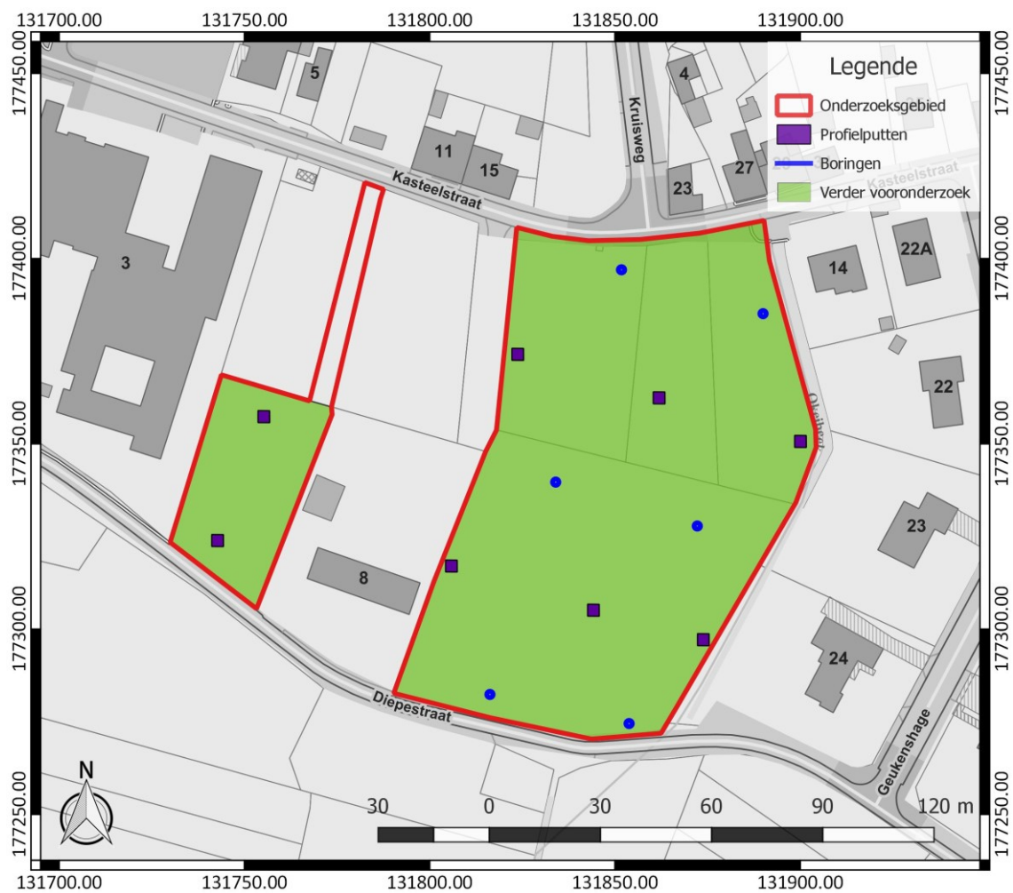
Figuur 3: Inplanting van de landschappelijke boringen (blauw) en de profielputten (groen), weergegeven op het GRB
