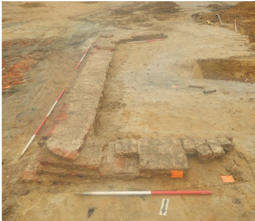
Figuur 3: S6091, zicht vanuit het noorden
