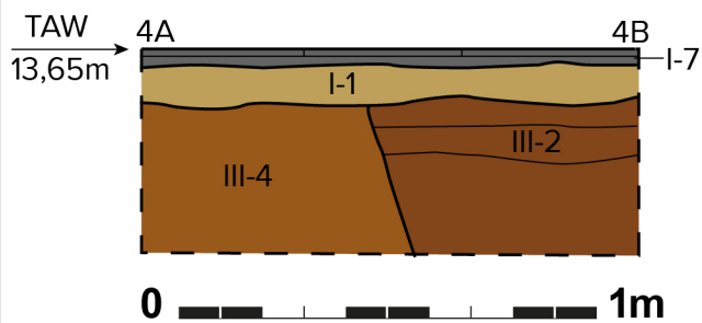
III - PROFIEL 4AB
