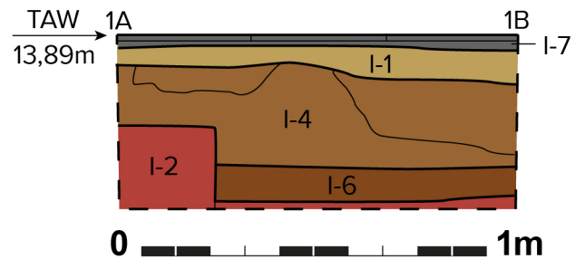
I - PROFIEL 1AB
