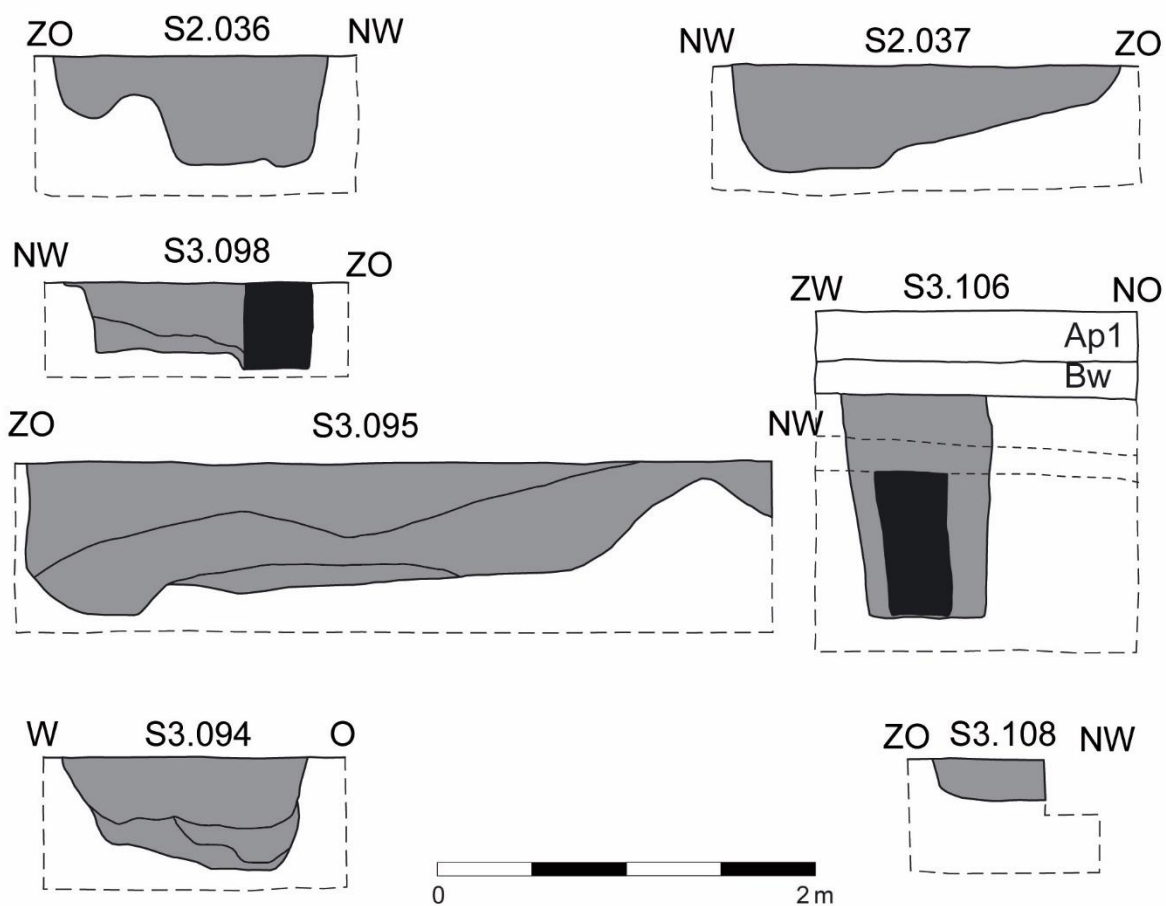
Figuur 17: Structuur H6 in vlak (schaal 1:200) en de coupetekeningen van de sporen (schaal 1:20).
