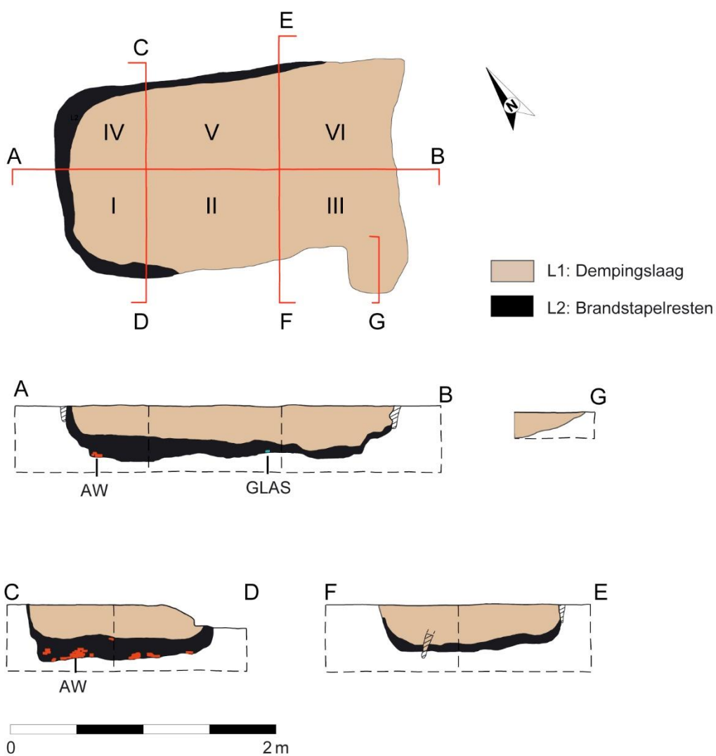
Figuur 35: Grondplan (schaal 1: 200) en coupes (schaal 1: 40) van brandrestengraf S1.091.
