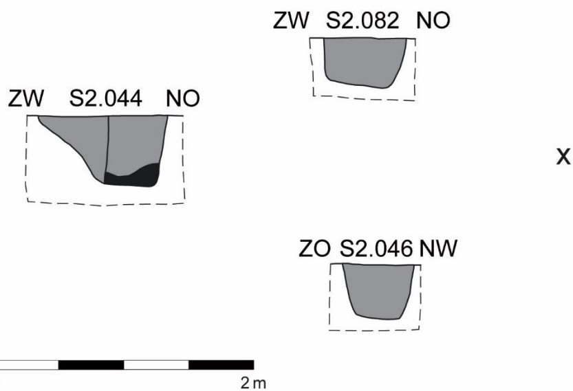
Figuur 23: Structuur H8 in vlak (schaal 1:200) met de coupetekeningen van de sporen (schaal 1:20).
