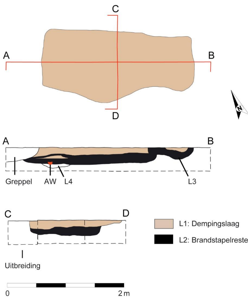
Figuur 32: Grondplan (schaal 1: 200) en coupes (schaal 1: 40) van brandrestengraf S1.067.
