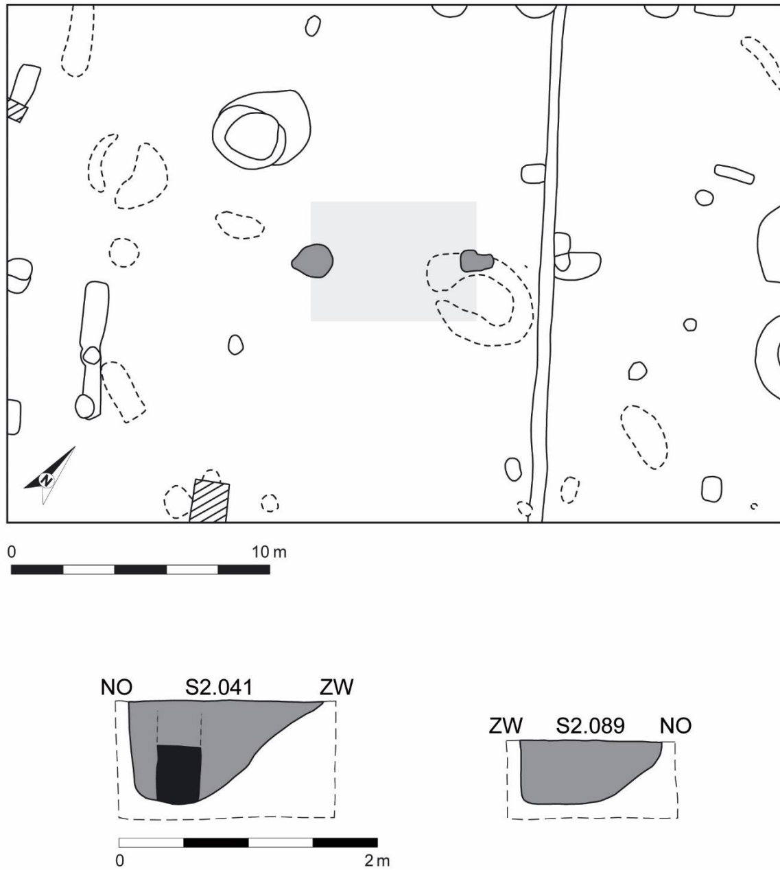
Figuur 8: Structuur H3 in vlak (schaal 1:200) en de coupetekeningen van de sporen (schaal 1:20).
