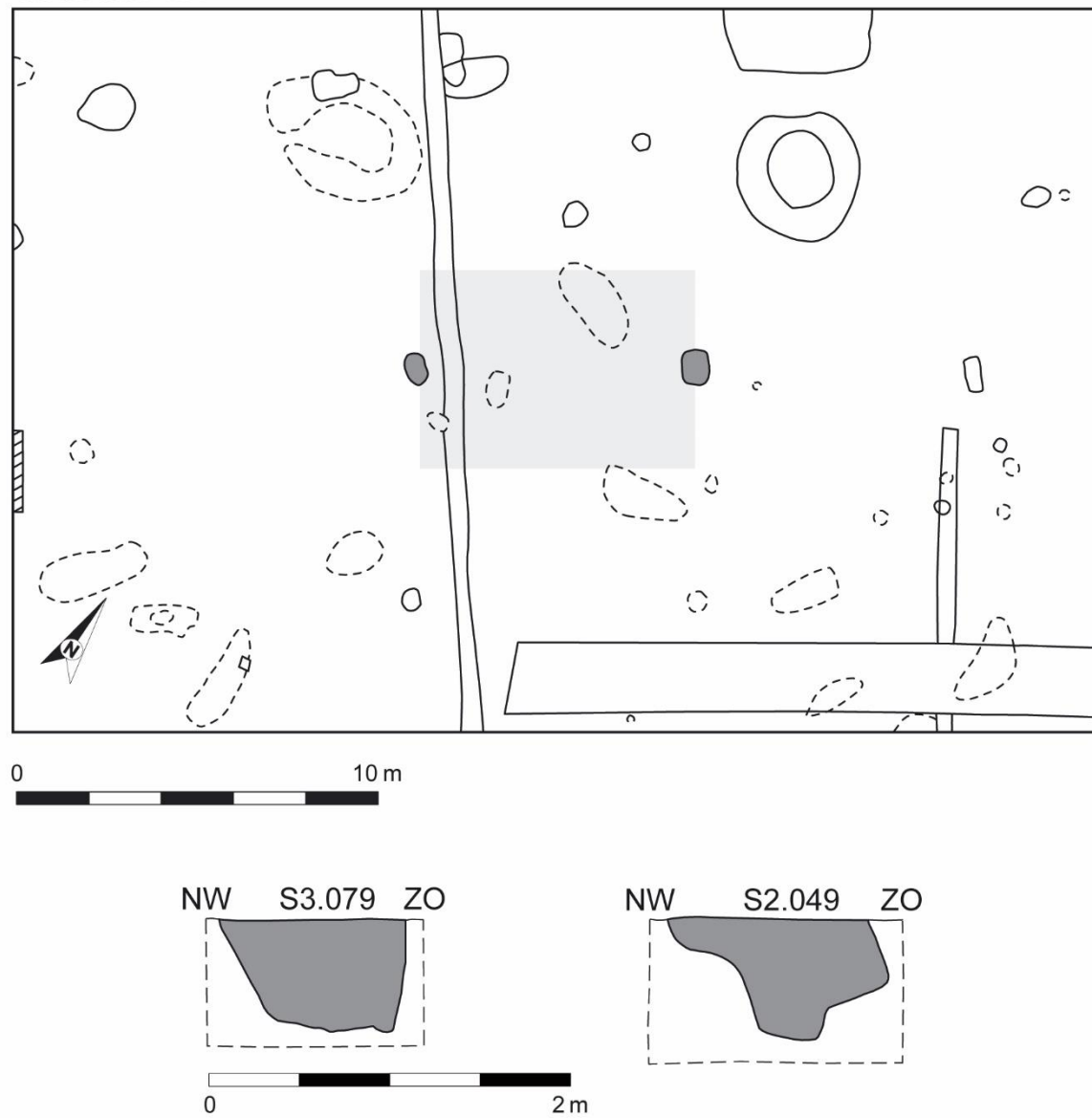
Figuur 11: Structuur H4 in vlak (schaal 1:200) en de coupetekeningen van de sporen (schaal 1:20).
