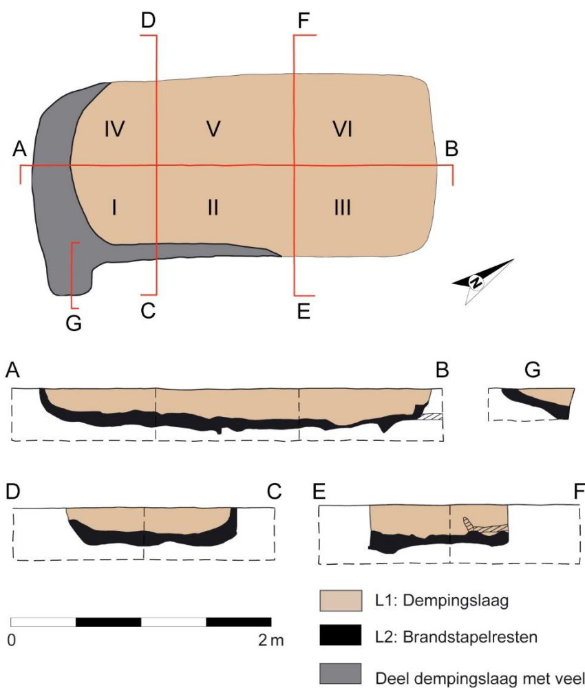
Figuur 38: Grondplan (schaal 1: 200) en coupes (schaal 1: 40) van brandrestengraf S5.009.
