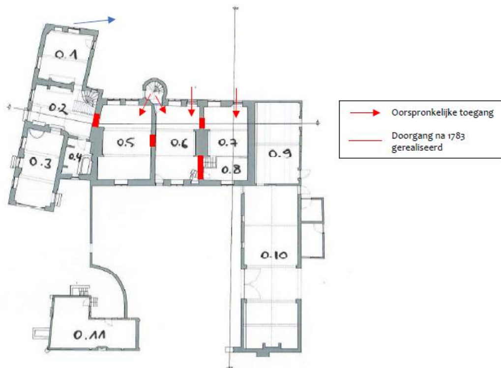
Figuur 4: Plan van de gelijkvloerse verdieping met ruimtenummering 15
