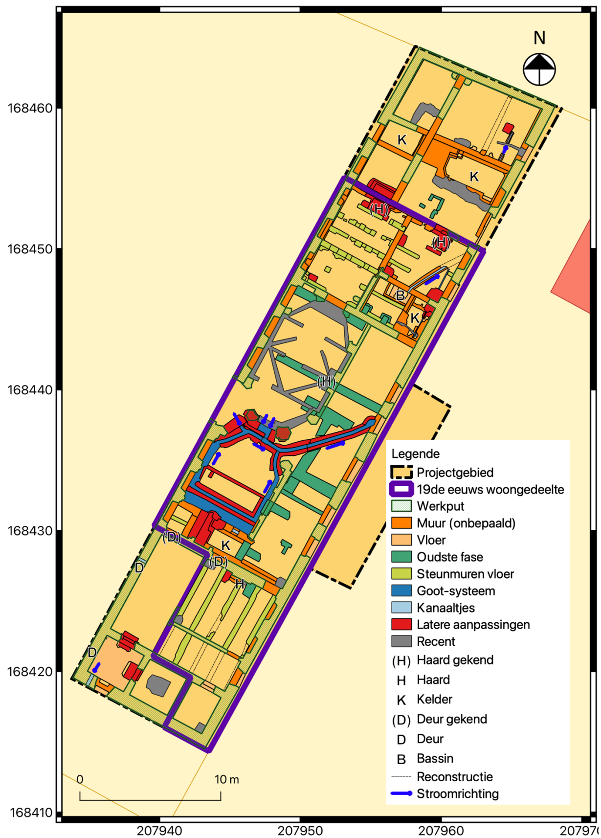
Fig. 3.52: Faseringsplan opgraving.
