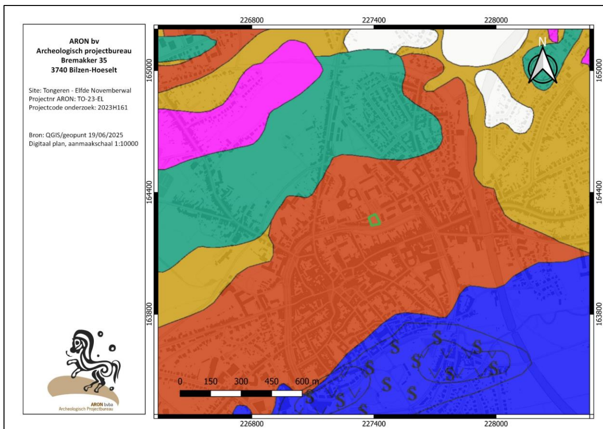
Afb. 9: Detail uit de Quartair profieltypekaart kaartblad 34-35 Tongeren met afbakening van het projectgebied (lichtgroen), het leempakket van 4-10 m dik (oranjebruin), het leempakket van 1-4 m dik (oker), het Jekeralluvium (blauw) en zandige leem (groen).
