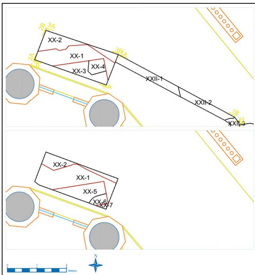
Figuur 110. Overzicht van de grondplannen van zone XX. Van links naar rechts en van boven naar onder: A, B.
