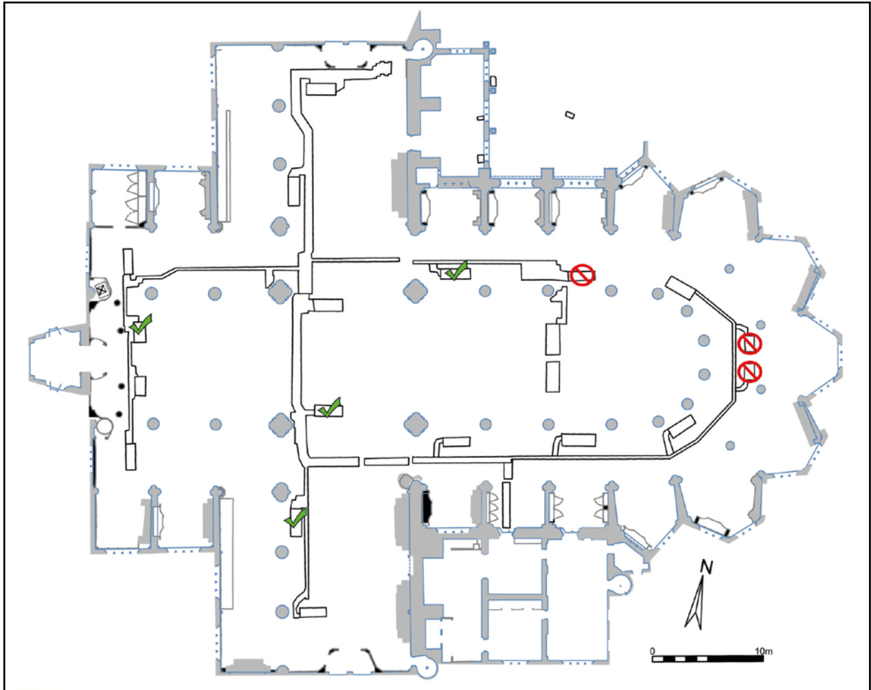
Figuur 30. Sleuvenplan met overzicht van de geslaagde en de niet geslaagde boringen
